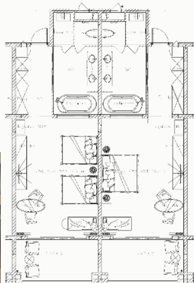
TYPE-A-1a 普通套房 56 m 2
